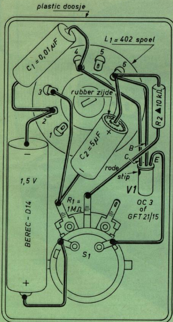
fig. 2. onderaanzicht v.h. gemonteerde apparaatje
